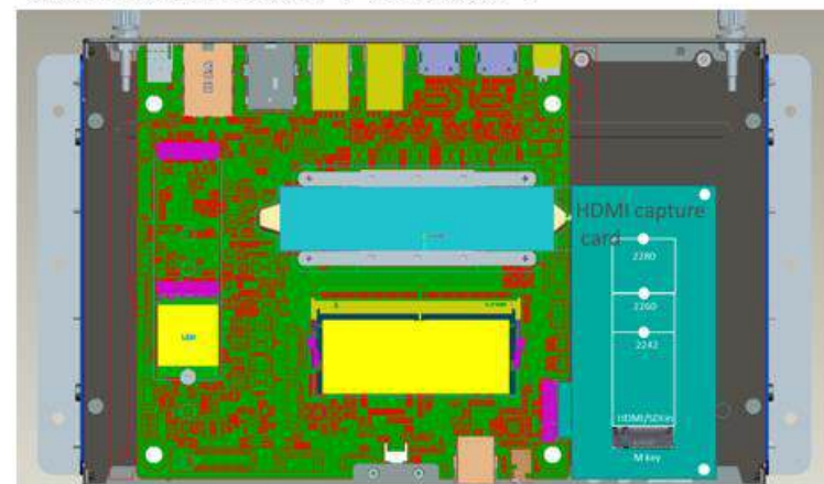
模組化設計：主機板 + HDMI擷取卡
